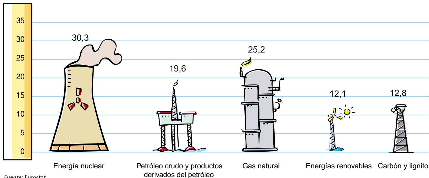
Producción de energía primaria en EU-15, porcentaje por fuente, 2001
