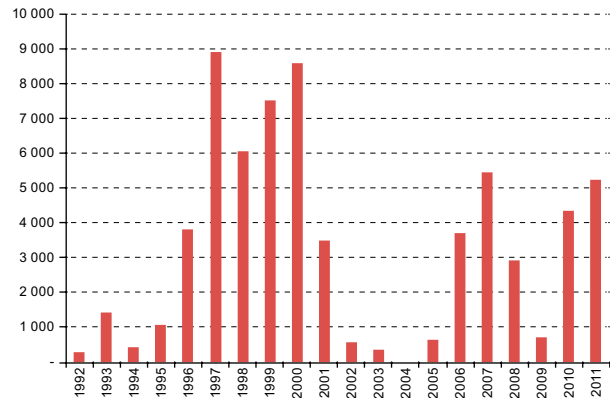
Gráfico IV.3 AMÉRICA LATINA: MONTOS TOTALES DE FUSIONES Y ADQUISICIONES TRANSFRONTERIZAS EN EL SECTOR ELÉCTRICO, 1992-2011 (En millones de dólares)
