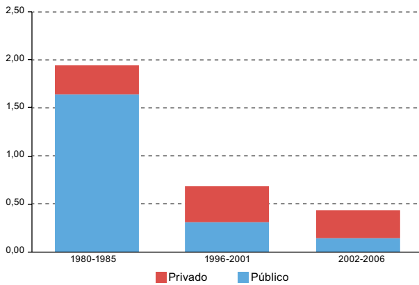
Gráfico IV.2 AMÉRICA LATINA (PAÍSES SELECCIONADOS): INVERSIÓN EN INFRAESTRUCTURA DE ENERGÍA, 1980-1985, 1996-2001 Y 2002-2006 a (En porcentajes del PIB)
