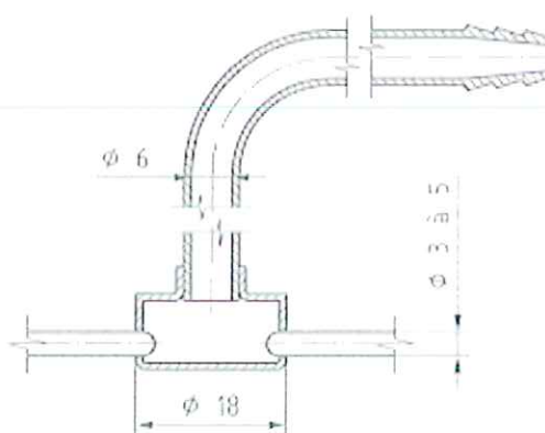
Figura 4 Sonda de toma de muestras para las chimeneas de ensayos de diámetros superiores o iguales a DN 100
